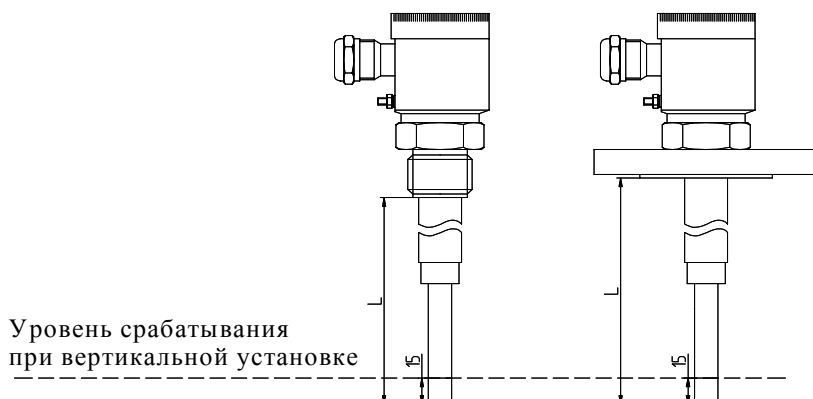
Рис. 1. Определение длины сигнализатора при различных типах присоединения.
